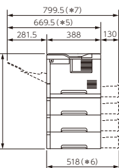
<側面図>
