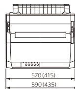
<上面図>
