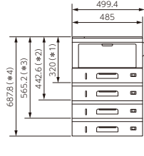
<正面図>
