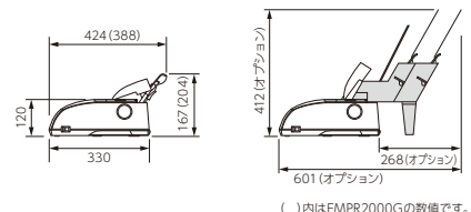
<側面図>
