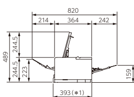
<側面図>
