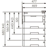
<正面図>
