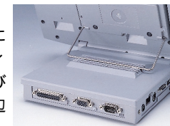
【ポータリプリケータ背面】
